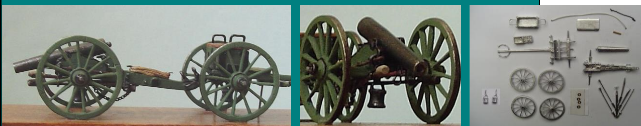
12 - pdr. Napoleon Gun, Confederate Typ, Geschütz mit Protze
